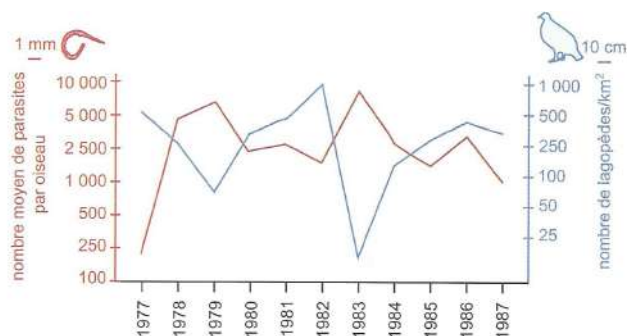
Relation entre la charge parasitaire moyenne et la densité des populations du lagopède d'Ecosse.
