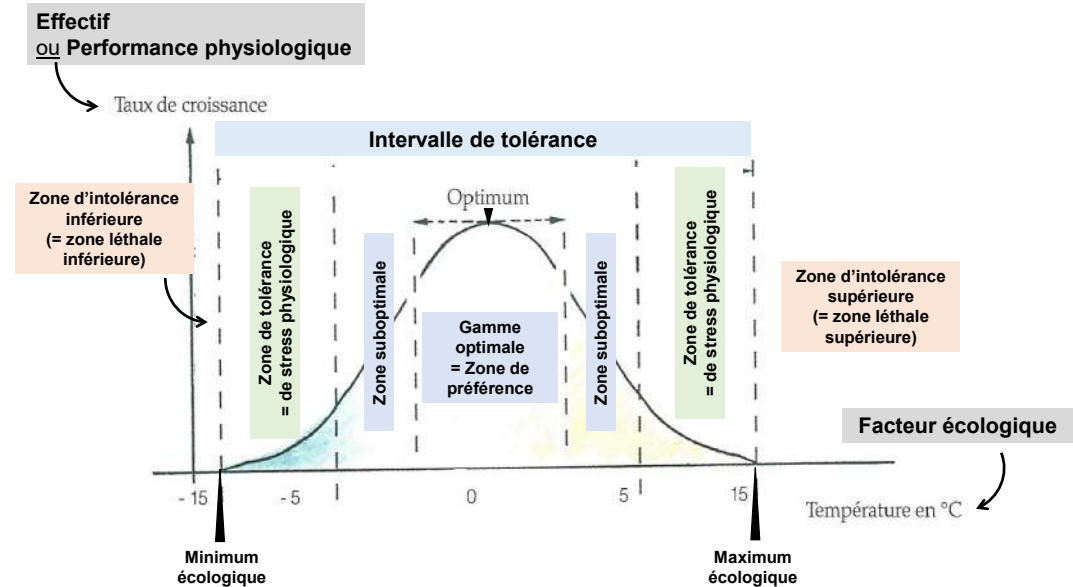
▲ FIGURE 80. Courbe de tolérance . D'après DUPUIS & FISCHESSE-TATE (2007), modifié. [Il s'agit ici d'une courbe de tolérance de la température par la Puce des glaciers, un Collembole vivant dans les sols enneigés]
