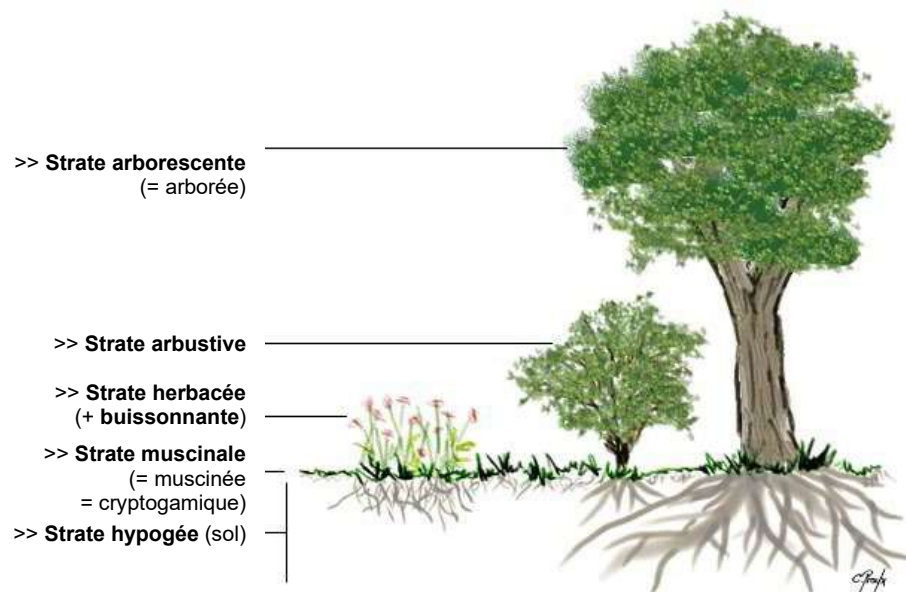
▲ FIGURE 5. Les strates végétales . https://lamaisondalzaz.wordpress.com/2010/11/01/lassociation-vegetale-un-revelateur/ (consultation mars 2018)
