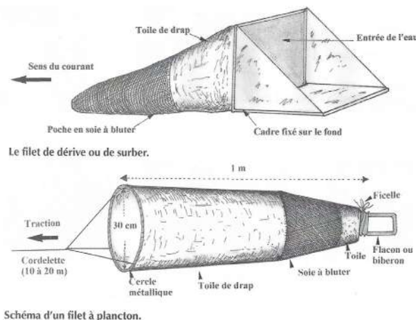
▲ FIGURE e. Quelques dispositifs de prélèvement en milieu aquatique. D'après FAURIE et al. (2002).
