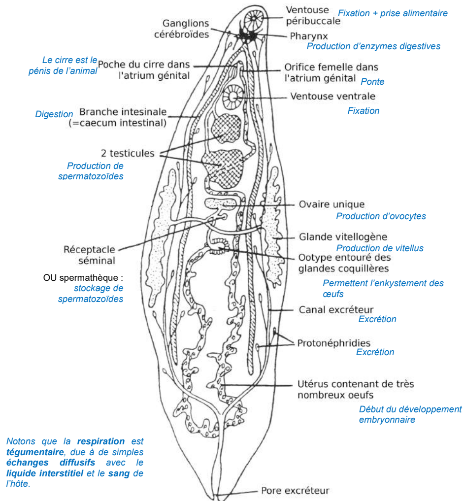
▲ FIGURE 105. Adulte de Dicrocoelium dentriticum . Taille : 6-10 mm par 2-3 mm. Document F. SAURETY (LEGTA Clermont-Ferrand Marmillhat).
