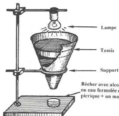
■ Extracteur de Berlèse.
