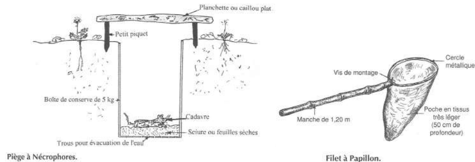
▲ FIGURE d. Un exemple de piège à insectes nécrophores (à gauche) et un filet à insectes pour la chasse à vue (à droite). D'après FAURIE et al. (2002).
