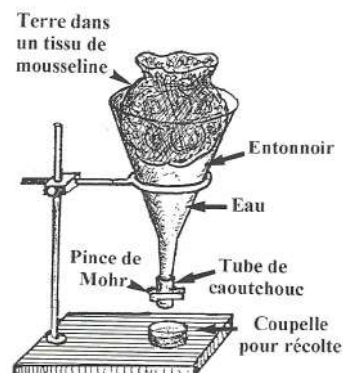
■ Extracteur de Bærmann.
