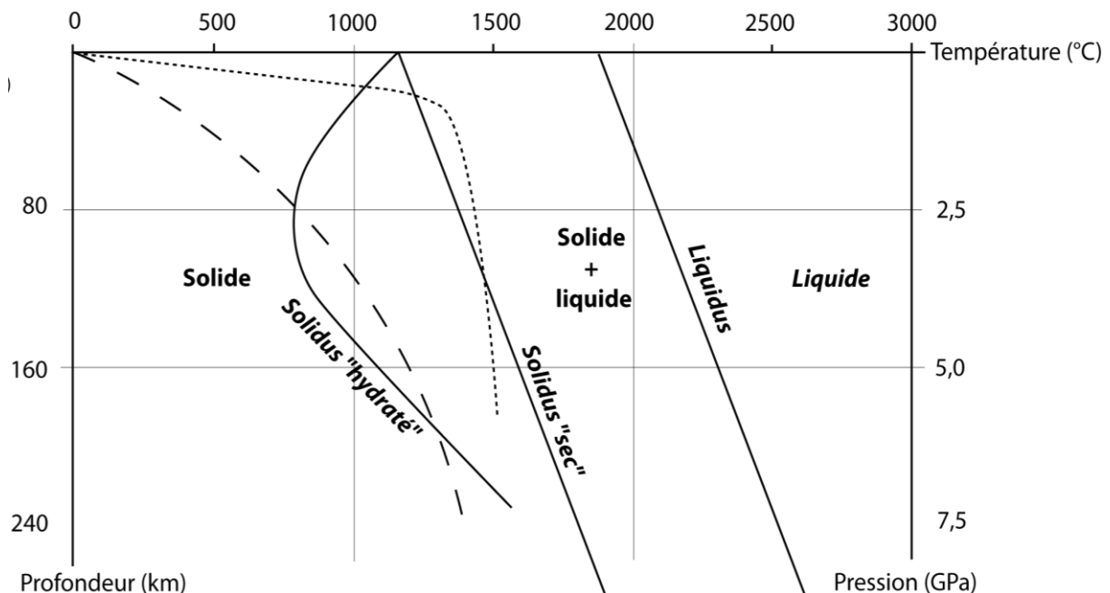
Document 6 - Diagramme Pression Température (PT) et fusion partielle hydratée de la péridotite
