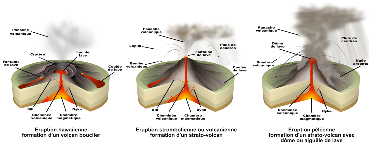
Document 1. Trois types d'éruptions associées à trois types d'édifice volcaniques.
