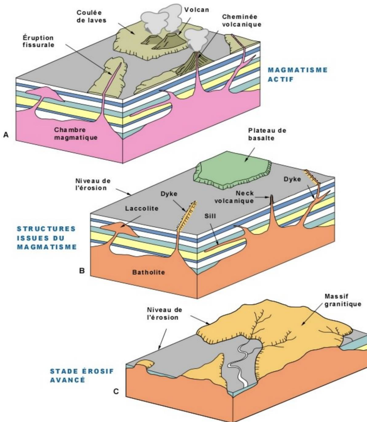
Document 3. Principales structures volcaniques et plutoniques, en cours d'activité (haut), après solidification et érosion faible (milieu, après ~10 000 ans), après érosion forte (bas, après ~10 Ma). Source inconnue, et c'est bien dommage !
