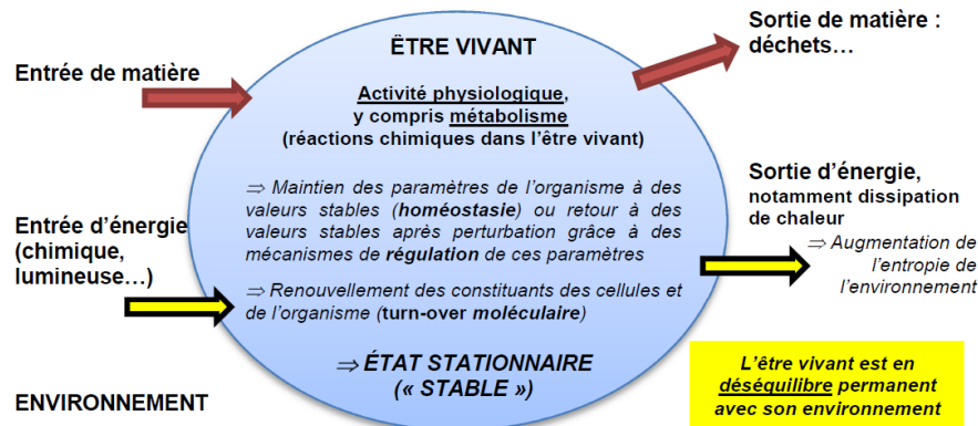
▲ FIGURE 2. Les êtres vivants, des systèmes thermodynamiques ouverts (= qui échangent de la matière et de l'énergie avec leur environnement). Voir le texte.
